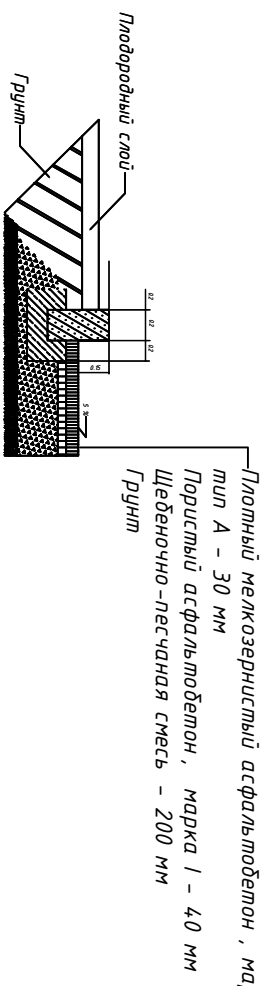
Схема дорожной конструкции, Тип 2
